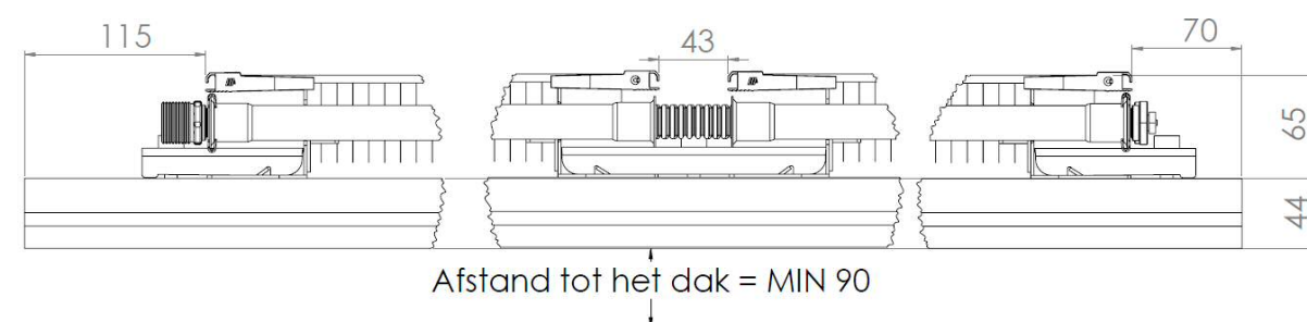
Figuur 6 - links afgebeeld de aansluitplug met 3/4" buitendraad, in het midden de tussenslang, rechts de eindplug met ontluchter – alle aansluiting zijn universeel en kunnen gespiegeld worden
