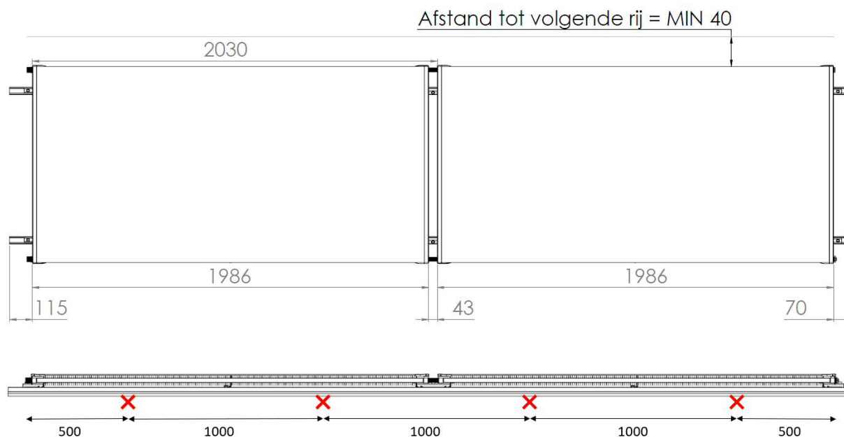
Figuur 3 – Afmetingen XL warmtepomppaneel, dakhaak of dakvoet plaatsing aangegeven met X
