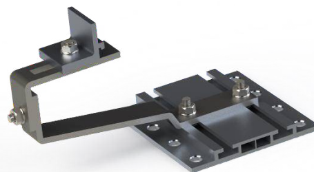
Figuur 2 - Triple Solar instelbare schroef-dakhaak
