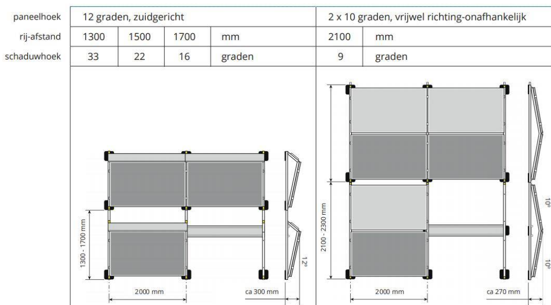
Figuur 3.2-a aanbevolen plat dak rijafstanden, bij type M2 360 200 landscape panelen
