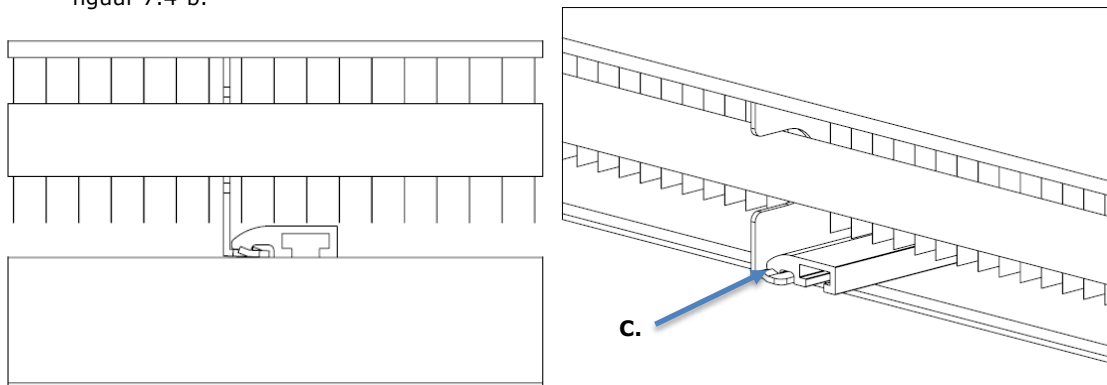
Figuur 7.3-b nokje omhoog buigen
