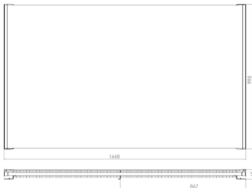
Figuur 2.1-b warmtepomppaneel type M2 300 200 landscape
