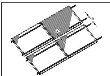
Figuur 5.1-d schuindak montage instructie dakankers (maten in mm).
