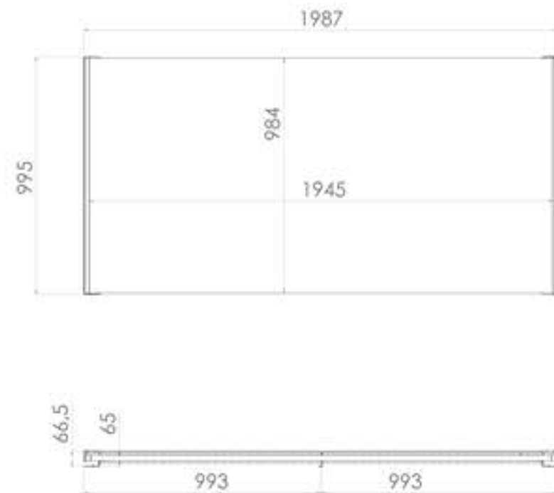
Figuur 2.1-a warmtepomppaneel type M2 360 200 landscape
